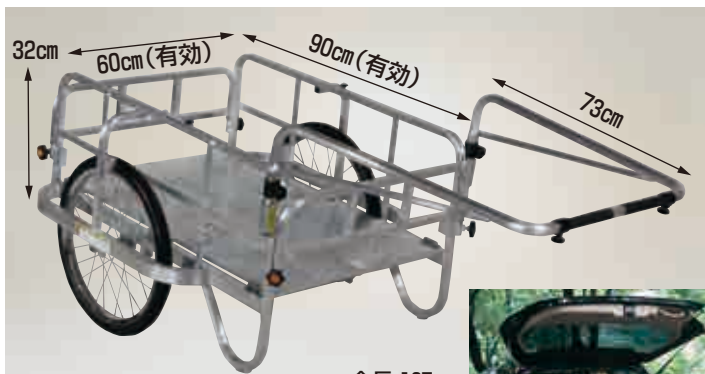
写真はHC-906
