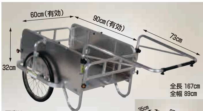
写真はHC-906A
