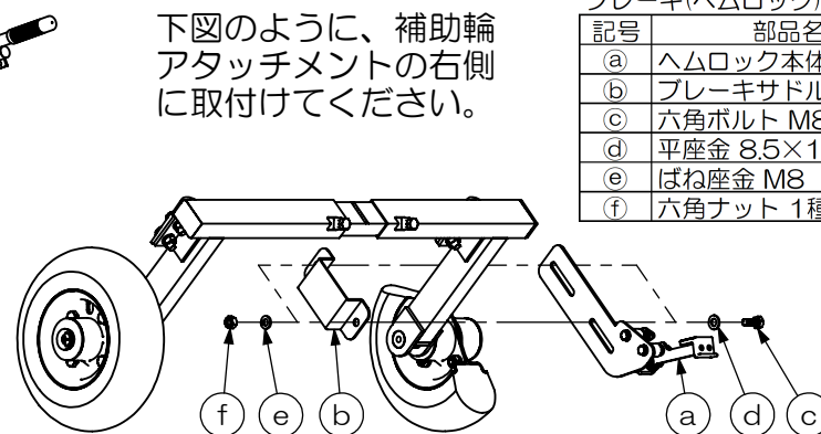
ブレーキ(ハムロック) 部材一覧表
