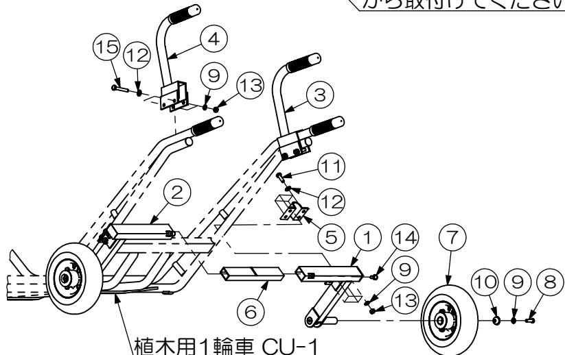
補助輪アタッチメント 部材一覧表
