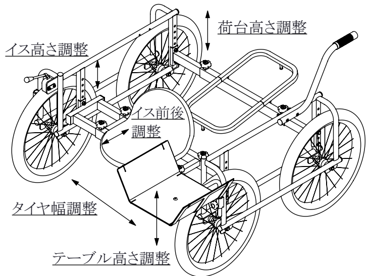
完成図
