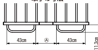
取手の寸法
