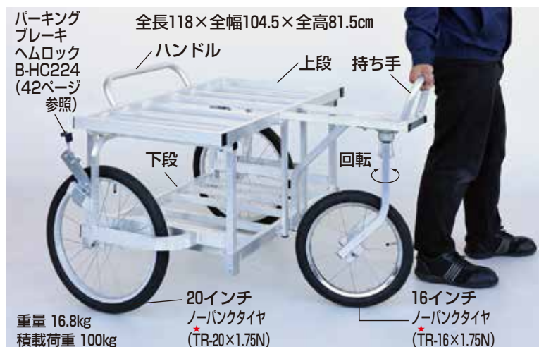
写真はTC-956NB
