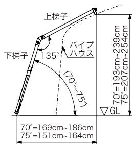
VHS-2500
