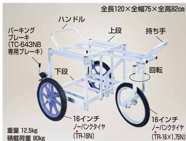
写真はTC-643NB
