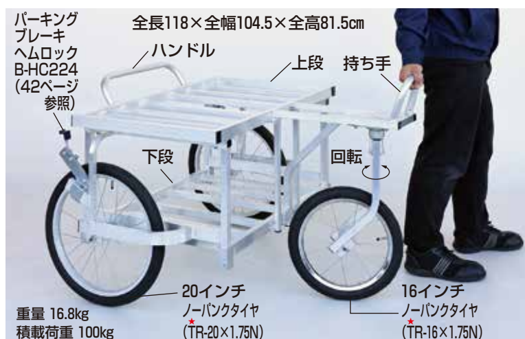
写真はTC-956NB
