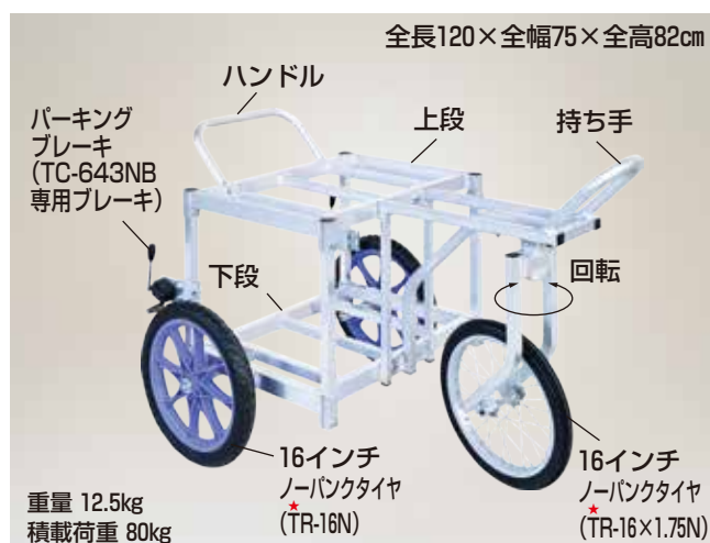
写真はTC-643NB
