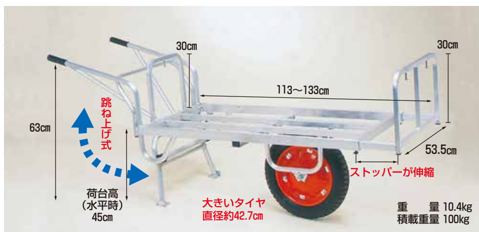
CN-65DU エアタイヤ * (TR-16×3DX) 定価 55,660円 (税抜 50,600円) (送料) 4台で元払い(離島は別途) (1台梱包)
