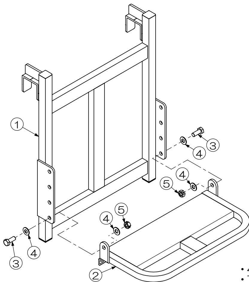
【組立説明図】 TS-540DW
